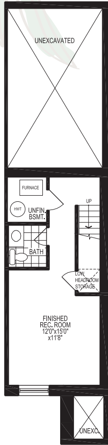
BASEMENT PLAN 'A' & 'B'
